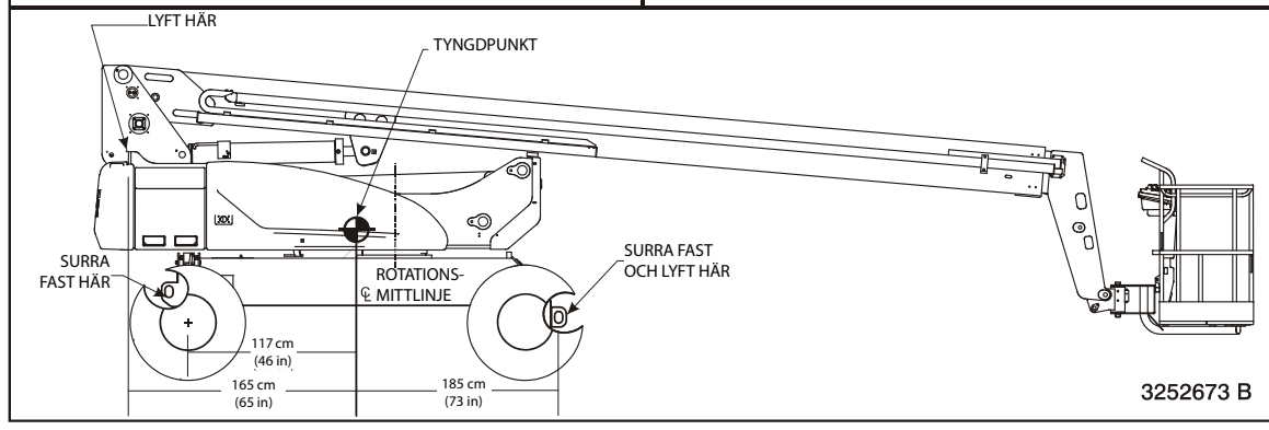
Fig. 4-5. Tabell över lyftning och fastsurning
