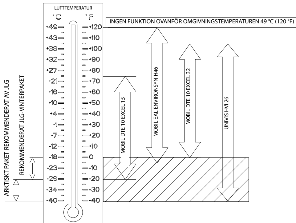
Fig. 7-1. Hydrauloljespecifikationer - blad 1 av 2
