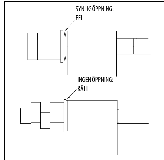
Fig. 6-2. Fastbultat externt fallskydd, vajer spänning
