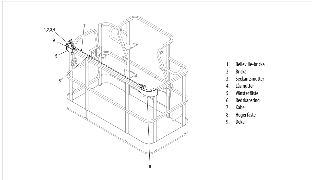
Fig. 6-3. Fastbultat externt fallskyddssystem
