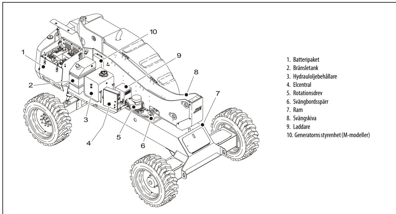
Fig. 2-1. Grundläggande nomenklatur - blad 1 av 3
